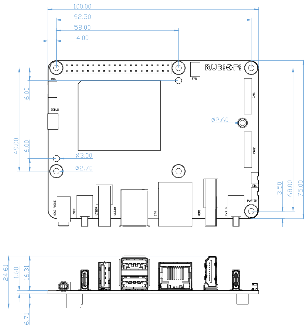
图 2-4. 魔方派 3 尺寸
