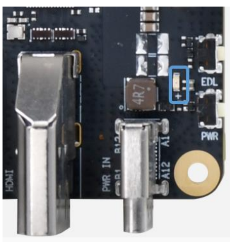
图 2-3. 电源指示灯
